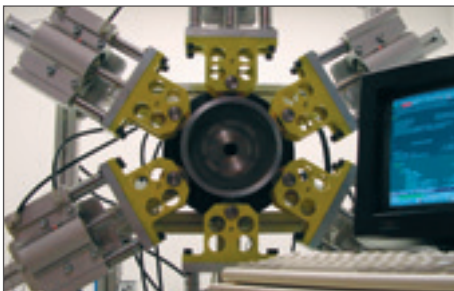
Görgő mérőpad
